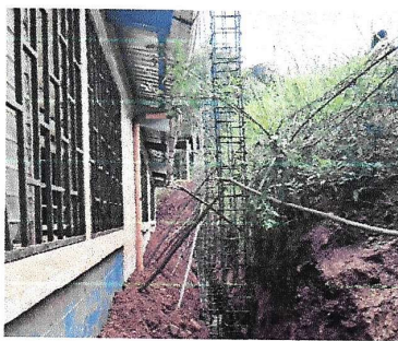
Foto 3: Parte de atrás del centro educativo donde se verifica el área a cubrir con la construcción del muro de contención.
