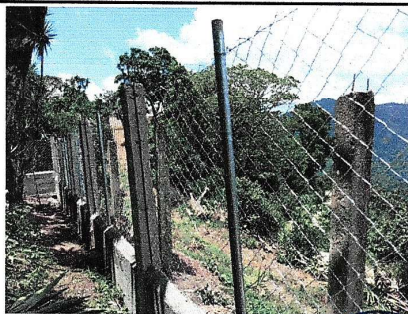
Foto 5: Malla colocada sobre cuatro hiladas de block intermedias y tubo galvanizado.
