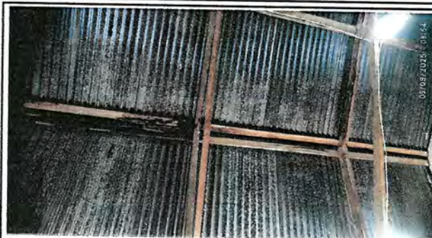
Foto 2: Sustitución de estructura de soporte de madera, por metal en aulas
