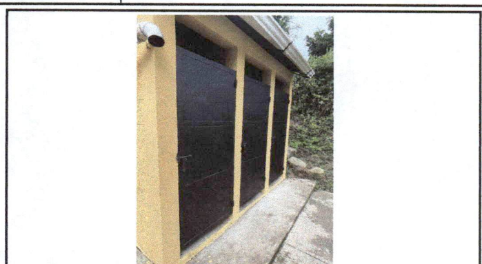
Foto 14: Fabricación e instalación de tres puertas de baños, medidas 0.80 x 1.80.
