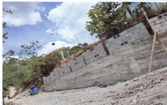
Sustitucion de muro por muro perimetral de cemento con piedra block de 20, tubo hg malla galvanizada soleras itermedias y columnas de hierro
