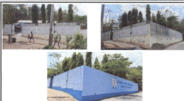
Foto 2: MURO PERIMETRAL. REPARACIÓN DE MURO PERIMETRAL DE BLOCK, CON SOLERAS INTERMEDIAS Y COLUMNAS.
