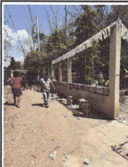
Foto 2: MURO PERIMETRAL. REPARACIÓN DE MURO PERIMETRAL DE BLOCK, CON SOLERAS INTERMEDIAS Y COLUMNAS.
