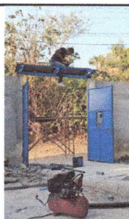
Foto 3: MANO DE OBRA ESPECIALIZADA (ALBAÑILERIA, HERRERIA, ELECTRICIDAD Y PLOMERÍA). FABRICACIÓN E INSTALACIÓN DE PORTÓN DE METAL DE INGRESO
