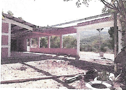
Foto 1: SEGUIMIENTO DE ESTRUCTURA METALICA Y CUBIERTA DE LAMINO A PATIO DE AULAS
