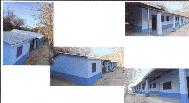
Foto 1: CUBIERTA DE LÁMINA. SUSTITUCIÓN DE LÁMINA, POR LÁMINA TROQUELADA ALUZINC CALIBRE 26; (DESMONTAJE Y MONTAJE).
