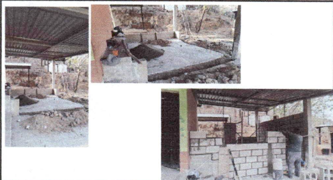
Foto 3: MURO DE PERIMETRAL (AULA). REPARACIÓN DE MURO PERIMETRAL DE BLOCK ( CONTINUACION DE MURO DE AULA BLOQUE III, CON REPELLO EN MURO INTERIOR Y EXTERIOR ). SE HICIERON CIMIENTOS CON ZAPATAS NUEVOS, YA QUE LO QUE ESTABA HECHO ESTABA INSEGURO Y SE CAYÓ AL INICIAR A TRABAJAR.
