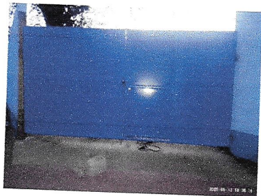
Foto 5: MANO DE OBRA ESPECIALIZADA (HERRERÍA). FABRICACIÓN E INSTALACIÓN DE PORTÓN DE METAL DE INGRESO AL ESTABLECIMIENTO EDUCATIVO (4.10 X 2.20 MTS.)
