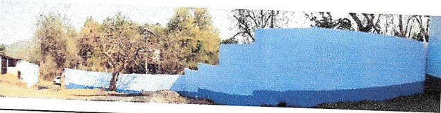
Foto1: MUROS PERIMETRAL. REPARACIÓN DE MURO PERIMETRAL DE BLOCK CON SOLERAS INTERMEDIAS Y COLUMNAS.
