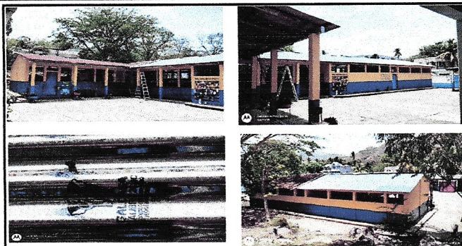
Foto1: CUBIERTA DE LÁMINA. SUSTITUCIÓN DE LÁMINA POR LÁMINA ACANALADA CALIBRE 26, INSTALADA.
