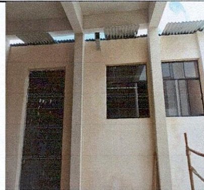
Foto 4: colocación de canal con dos costaneras legitimo.
