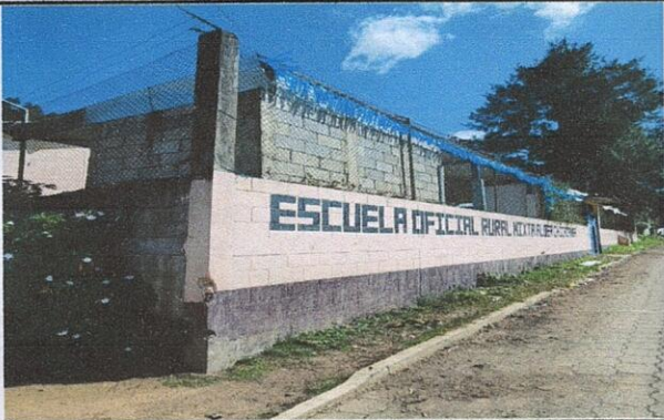
Foto 1: FRENTE LADO IZQUIERDO DEL MURO PERIMETRAL, EN ESTE LADO SE CONTINUARÁ CON EL MURO PERIMETRAL 2 METROS MÁS HACIA ARRIBA. SERÁN 17 MTS DE LARGO POR 2 MTS DE ALTO MÁS PARA HACER UN TOTAL DE 34 MTS CUADRADOS.
