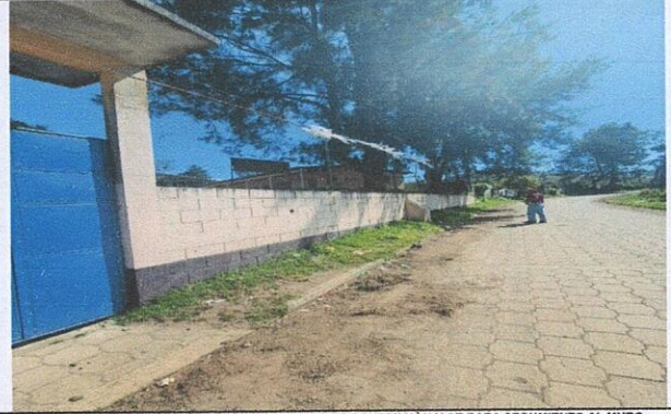
Foto 2: FRENTE LADO DERECHO MEJORAMIENTO DEL MURO DE CONTENCIÓN Y SE DARÁ SEGUIMIENTO AL MURO PERIMETRAL.
