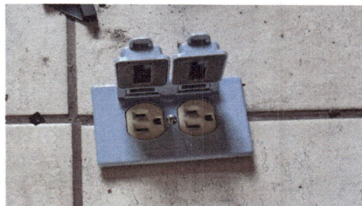
Foto 18: en la imagen se observan los tomacorrientes de piso ya reemplazados y correctamente instalados. Los nuevos dispositivos presentan una fijación adecuada y funcionamiento correcto
