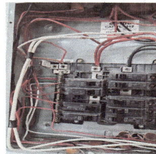
Foto 6: en la imagen se observa el tablero eléctrico tras concluir los trabajos de reparación. El cableado se aprecia correctamente organizado y asegurado, con las conexiones firmes en los interruptores. El sistema quedó en condiciones adecuadas para su correcto funcionamiento y uso.
