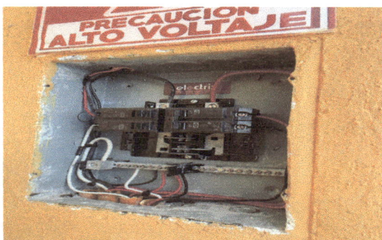
Foto 9: en la imagen se observa el tablero eléctrico tras concluir los trabajos de reparación. El cableado se aprecia correctamente organizado y asegurado, con las conexiones firmes en los interruptores. El sistema quedó en condiciones adecuadas para su correcto funcionamiento y uso.
