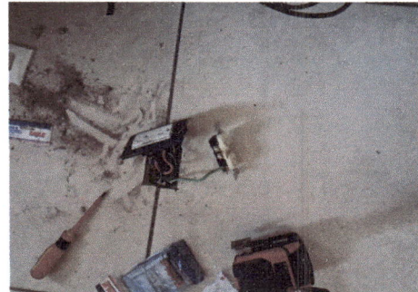
Foto 10: durante la actividad se instalan tomacorrientes de piso, garantizando una distribución eléctrica funcional para el área
