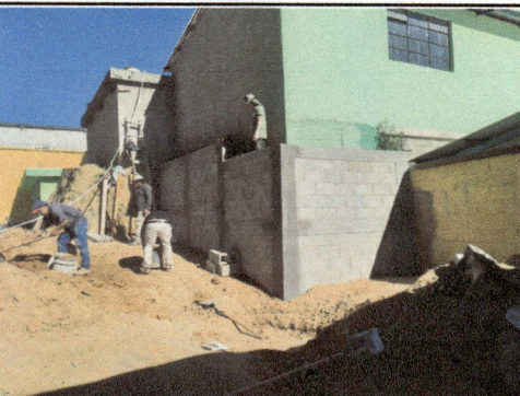
Foto 5: Muro de contención segundo ambiente reubicando tierra y rellenado en donde es necesario.
