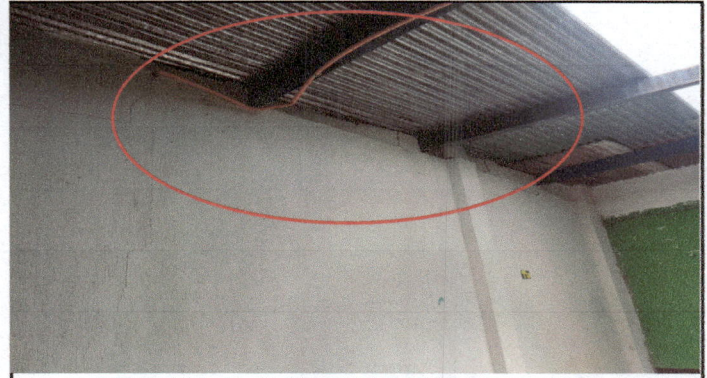
Foto 2: Grietas que muestran el desplome de la pared (primer ambiente)
