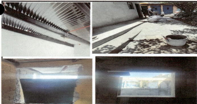
Foto 5: Instalación eléctrica, remodelación y fundición de pavimento del corredor de la cocina, demolición por apertura de puertas y cierre de ventana
