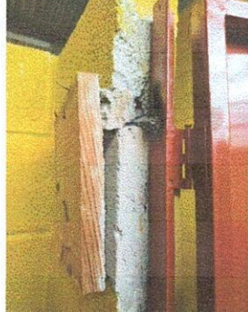
Foto 3: En los servicios sanitarios se le realizara trabajos de reforzamiento en los pines de los servicios sanitario ya que algunas puertas estan por caerse.
