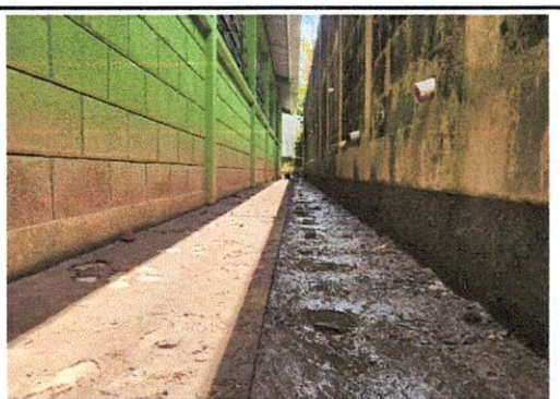
Foto 6: La saturación de humedad en el suelo superior pone en riesgo los salones de clase que el muro se caiga.
