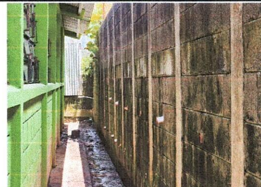
Foto 4: El muro de contención está pandeado, la humedad de la tierra está sobrecargando el muro de contención.
