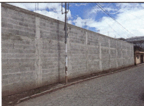
FOTO 9: SOLERA E CORONA EN EL MURO PERIMETRAL
