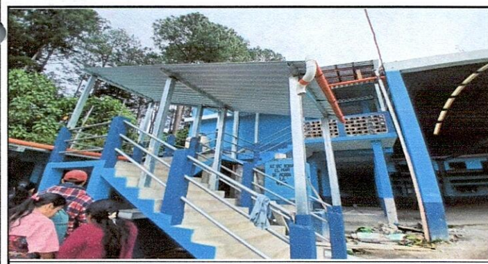
Foto 5: estructura de techo con estructura metálica en gradas del segundo al primer nivel con bajadas de agua.
