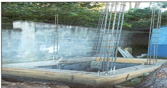
Foto 4: Levantado de muro para implementación de sanitarios.
