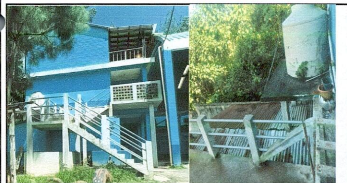
Foto 5: estructura de techo en gradas del segundo al primer nivel, motivo es que en tiempo de lluvia los jóvenes se mojan cuando van al sanitario.
