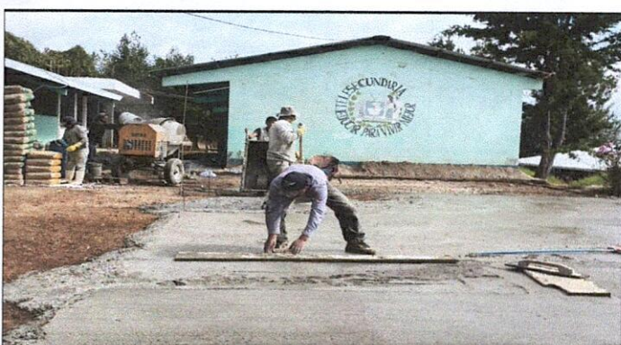
Foto 4: LOSA DE PATIO: ELABORACIÓN DE PLANCHAS DE CONCRETO
