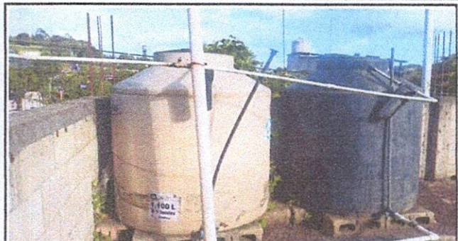
Foto 8: SUSTITUCIÓN DE DEPOSITOS DE AGUA
