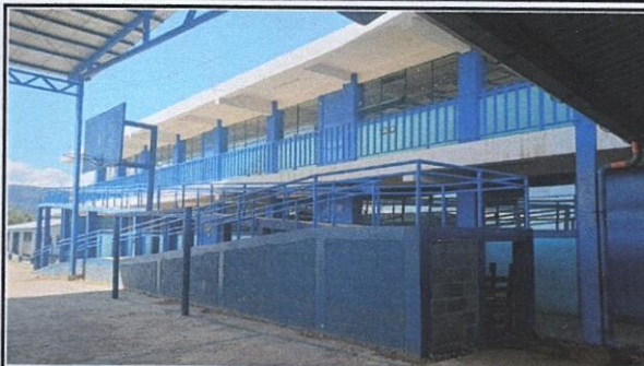
Foto 2: Modificación de rejas para rampa, las rejas actuales no cumplen con las medidas de seguridad necesarias.
