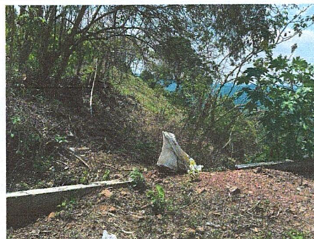
Foto 4: Este muro es la parte derecha del establecimiento, tiene solo fundido la solera, por lo que, no tiene una seguridad para los niños, es por ello la necesidad de aumentar la altura de la pared con 5 hiladas de block y malla.
