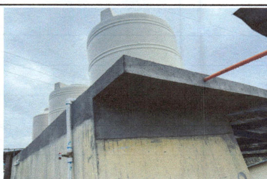
Foto 6: Construcción de loza para dos tinacos
