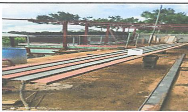
Foto 4: Se remodeló el techo de enfrente del establecimiento con estructura metálica, la cual se protegió con pintura anticorrosiva
