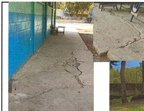
Foto 3: Sustitución de piso de torta de concreto del corredor de los salones de clases 148 m2 y muro de tension de 30 m2 al borde del piso.
