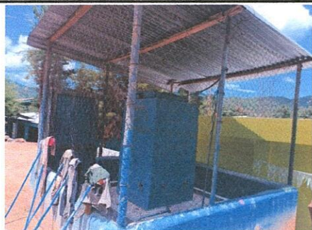
Foto 5: Suministro de Circulación de Pileta con instalación de Malla 25 m2
