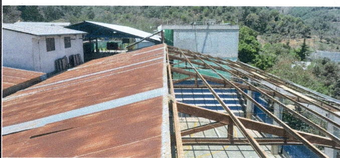
Foto 3: Avanzan trabajos de sustitución de lámina, se realiza el desmontaje total y se comienza a dar mantenimiento a estructura metálica
