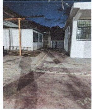
Foto 4: INSTALACION DE DRENAJE PLUVIAL DONDE SE RECOLECTARA AGUA PLUVIAL Y AGUA GRIS DE LAVAMANOS HACIA COLECTOR EXISTENTE.
