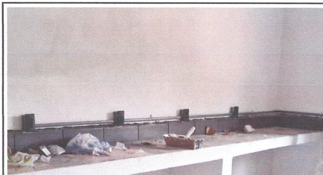
Foto 3: INSTALACIÓN DE TUBERÍA Y TOMACORRIENTES EXPUESTOS EN LABORATORIO DE BIOLOGÍA (Incluye instalación de cableado desde centro de carga).
