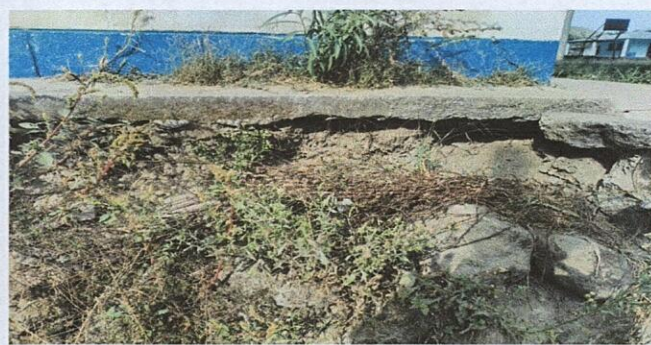
PROTECCION DE TALUD EN AULA A TRAVES DE MURO DE CONTENCIÓN CONSISTENTE EN: ELABORACION DE ZAPATA, CAITE, COLUMNAS, FUNDICIÓN DE COLUMNAS, LEVANTADO Y SISADO DE
