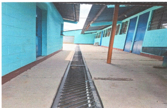
4. Reparación de cunetas de concreto: Consistente en elaboración de una cuneta de concreto y su respectiva tapa metálica.
