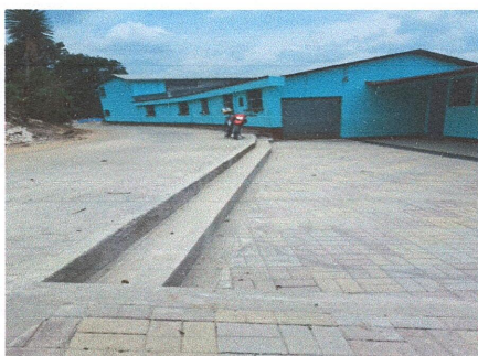
5. Repación de banquetas de concreto: Consistente en demolición del banquete de concreto actual, trazo y elaboración de nuevas gradas y elaboración de una rampa de ingreso e egreso en la escuela.
