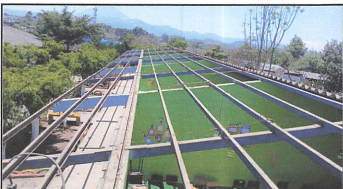
Foto 3: Avance en la colocación de lámina troquelada calibre 26. tomada en la parte superior de los salones .
