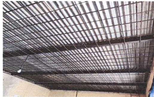
Instalación de 34 metros cuadrados de cielo falso fibra de cemento tipo colonial color blanco
