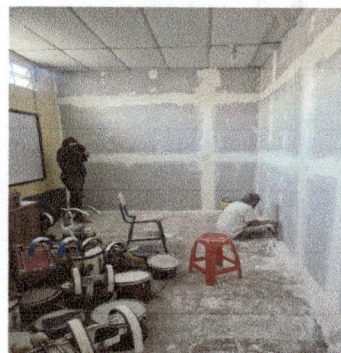
Foto 4: Terminado de división con tabla yeso por dentro.
