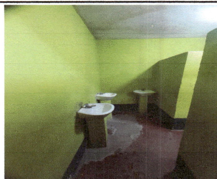
Foto 4: Instalación de piso antideslizante en baños, lavado de superficie con ácido muriático.
