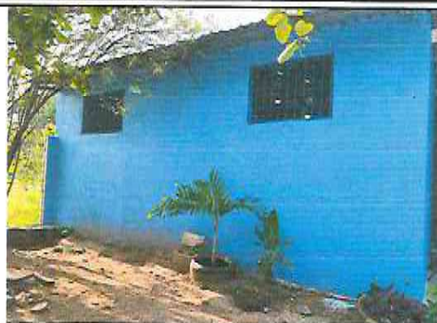
Foto 2: repello y cernido de paredes de salon de clases (exterior) terminado
