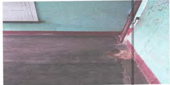
Foto 4: Reparación piso liquido por torta de concreto en aula no. 2
