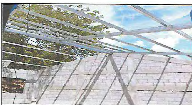
Foto 6: Sustrucción de estructura de soporte de madera, por metal en el aula.
