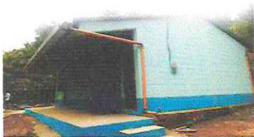
Foto 3: Sustitución de bajada de agua pluvial de tubo PVC de 3"
