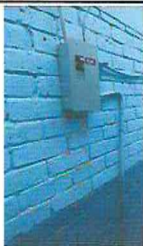
Caja de flipones, flipones y cableado nuevo instalado.
