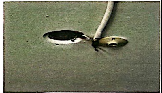
Foto 10: Sustrucción de plafoneras
