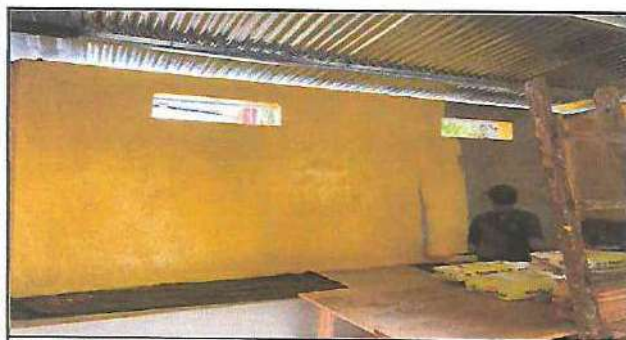
Foto 11: Módulo Cocina. Realizando aplicación de pintura en muros interior y exterior en terminado de cernido.
