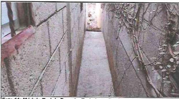
Foto 11: Módulo Red de Drenaje. Trabajo realizado en mantenimiento red de drenaje (reposición de tubería + reposición de concreto).
